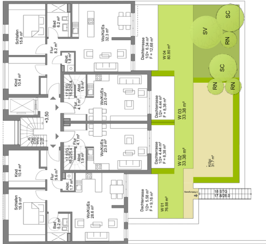
1. Obergeschoss
